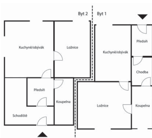
Sociální bydlení v lihovaru - přízemí
